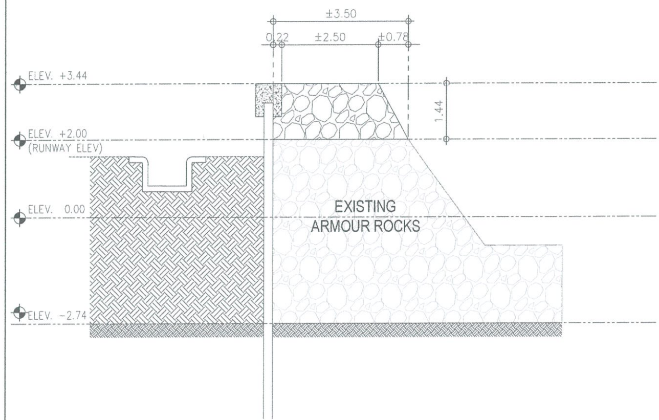
3 C-3 C-3 ARMOUR ROCKS @ STA. 0-140 DETAILED SECTION SCALE: 1:100 M
