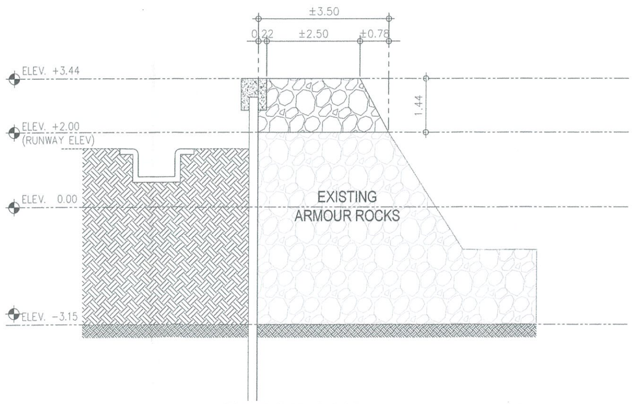
4 C-3 C-3 ARMOUR ROCKS @ STA. 0-120 DETAILED SECTION SCALE: 1:100 M
