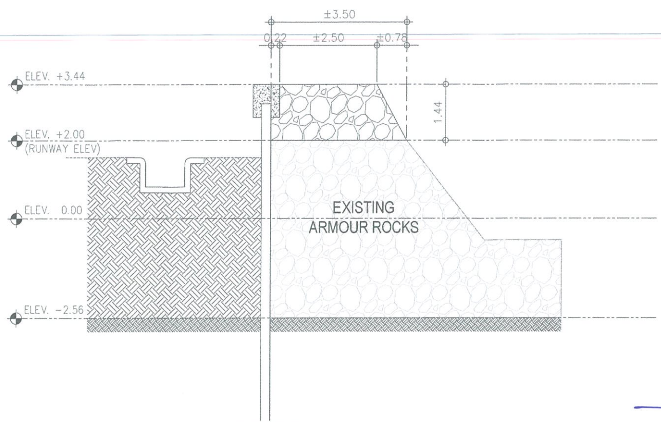
2 C-3 C-3 ARMOUR ROCKS @ STA. 0-160b DETAILED SECTION SCALE: 1:100 M
