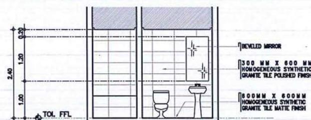
4 PWD TOILET @ LOBBY A-9 SCALE: 1 : 50 M
