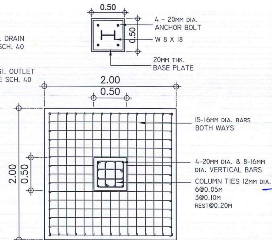
14 S-2 S-2 C1-F1 DETAIL SCALE: 1 : 35 M
