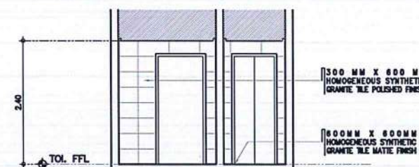
5 PWD TOILET @ LOBBY A-9 SCALE: 1 : 50 M
