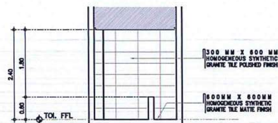
2 PWD TOILET @ LOBBY A-9 SCALE: 1 : 50 M
