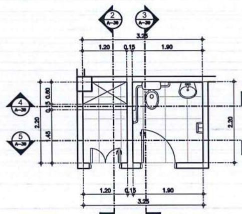
1 PWD TOILET @ LOBBY A-9 SCALE: 1 : 50 M
