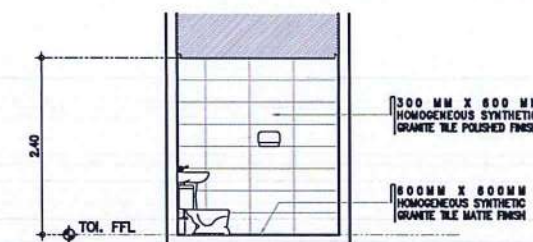
3 PWD TOILET @ LOBBY A-9 SCALE: 1 : 50 M
