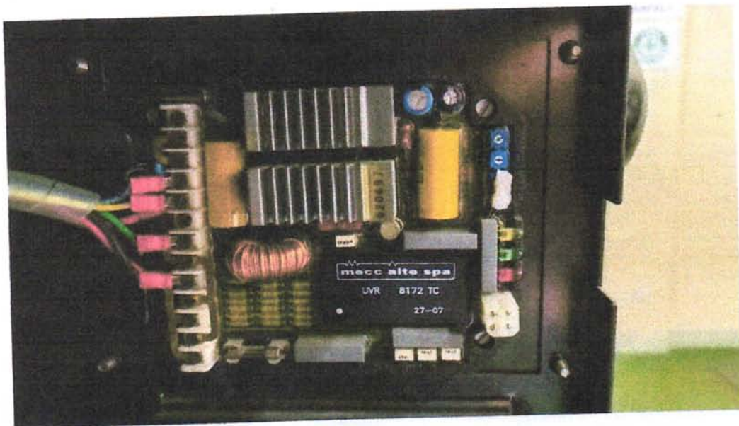
DEGS 2 AVR
